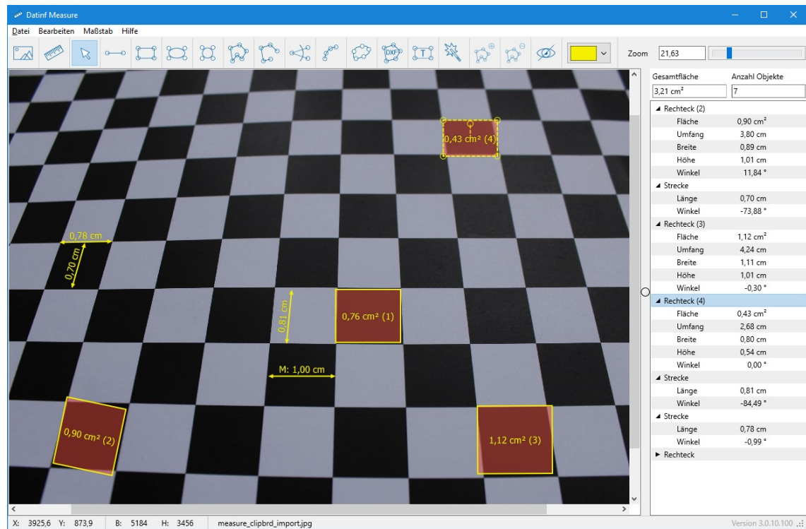
Abb. 11: Beispiel Messfehler durch Verzerrung - Aufnahmeabstand ca. 30 cm, Zoomeinstellung: Weitwinkel; erwartete Größe der Quadrate: 1 cm 2 , Messungen nicht sinnvoll möglich
