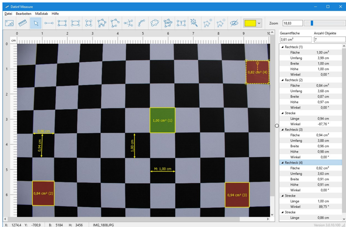
Abb. 10: Beispiel Messfehler durch Verzeichnung - Aufnahmeabstand ca. 30 cm, Zoomeinstellung: Weitwinkel; erwartete Größe der Quadrate: 1 cm 2 , gemessen im Randbereich: 0,84 cm 2
